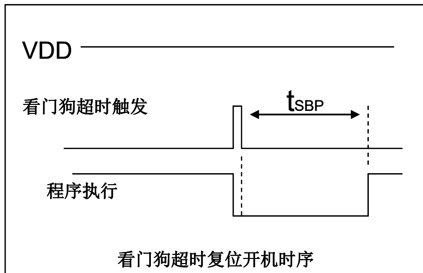
图 19: 看门狗超时溢出时序图
