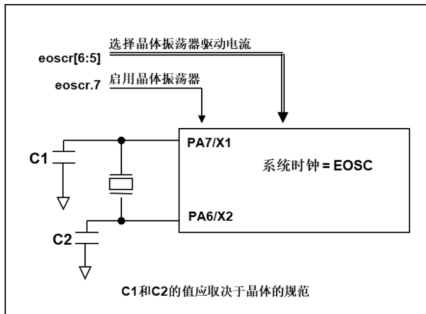
图 2: 晶体振荡器的硬件连接
