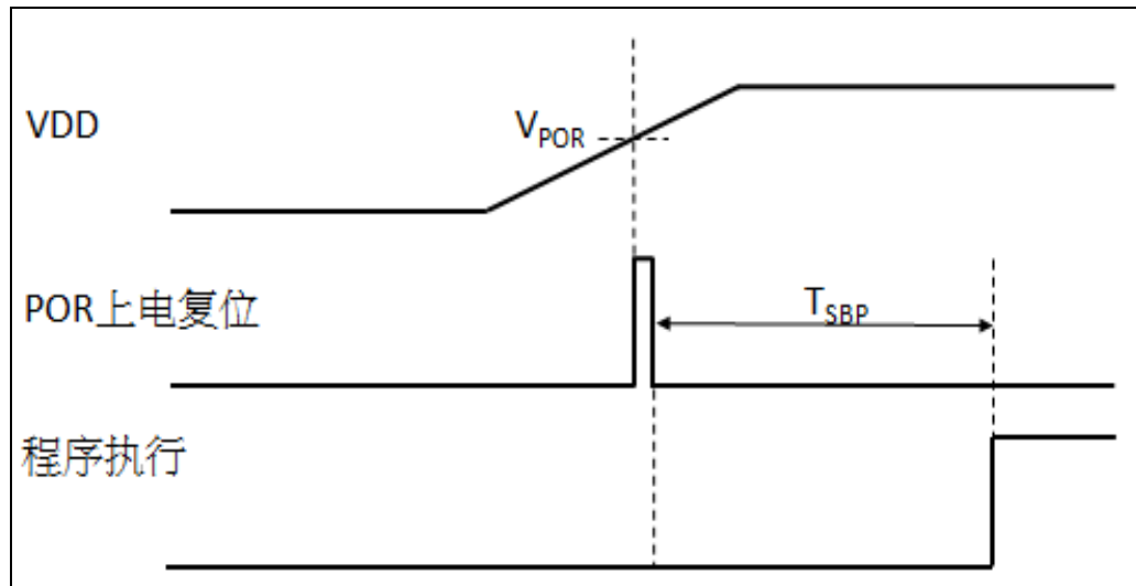
图 1：上电复位时序
